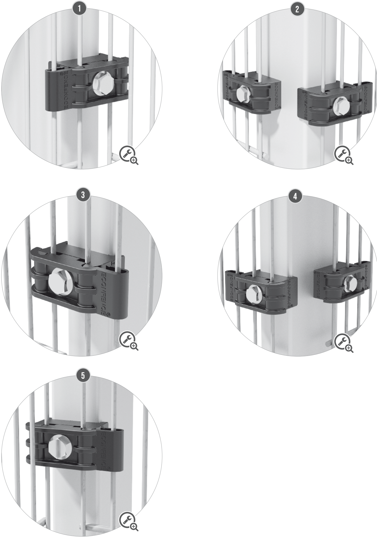
Widok gotowego zespołu elementów mocujących ZB31004
